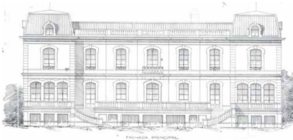
Palacio Munoa. Vista de conjunto principal (↑) y alzado de fachada principal (↓).
