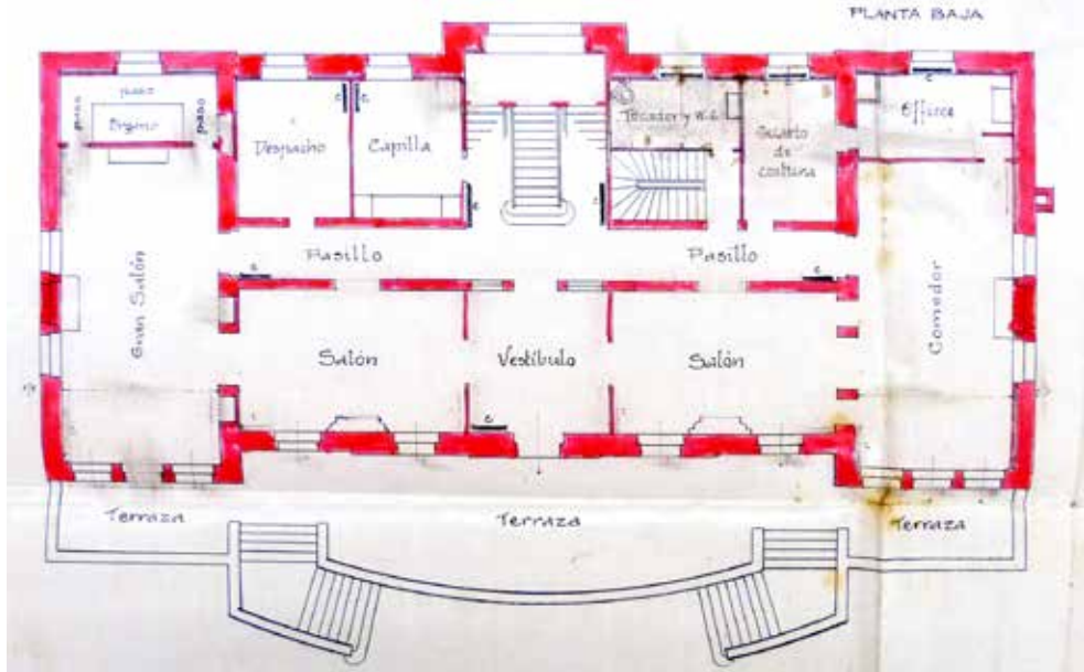
Palacio Munoa. Plantas de sótano y baja.
